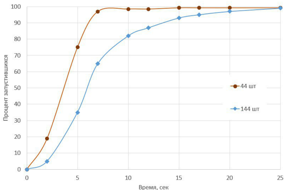
Рисунок 3 Задержка активации при одновременном групповом запуске Аврора-ДС-ПРО исп. Л
