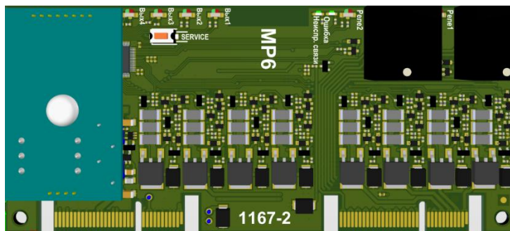
Рисунок 21 Внешний вид модуля MP6
