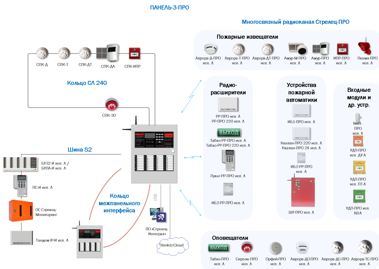
Рисунок 1 Система АППЗ на базе ППКУП Панель-3-ПРО исп. Л
