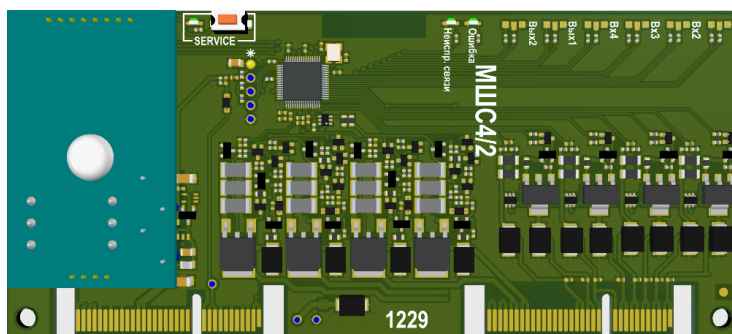
Рисунок 20 Внешний вид модуля МШС4/2
