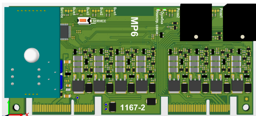
Рисунок 21 Внешний вид модуля MP6
