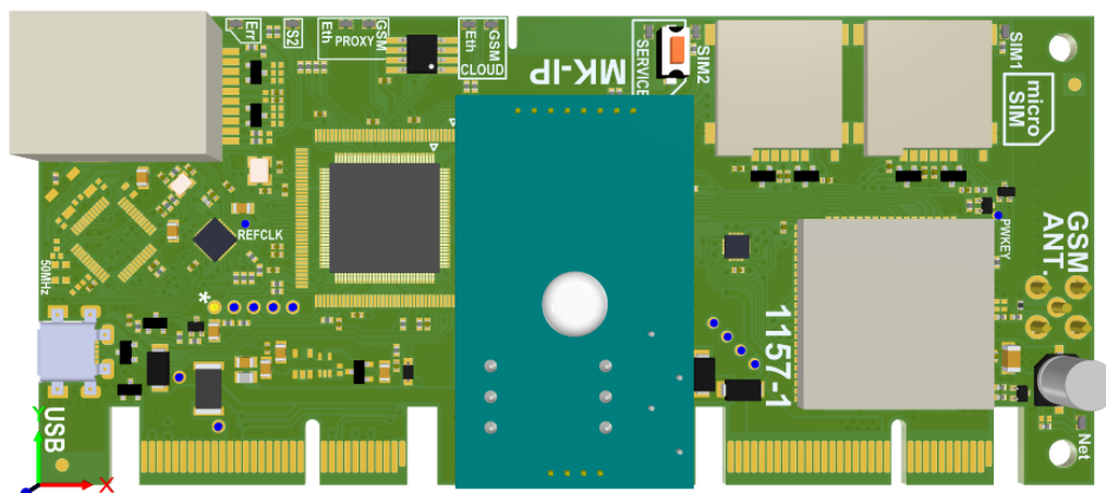
Рисунок 19 Внешний вид модуля МК-IP
