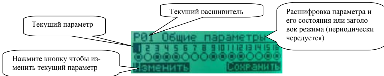
Рис.16 Программирование общих параметров расширителя
